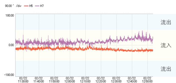
流入/流出判断的例(5次、7次谐波流入)
