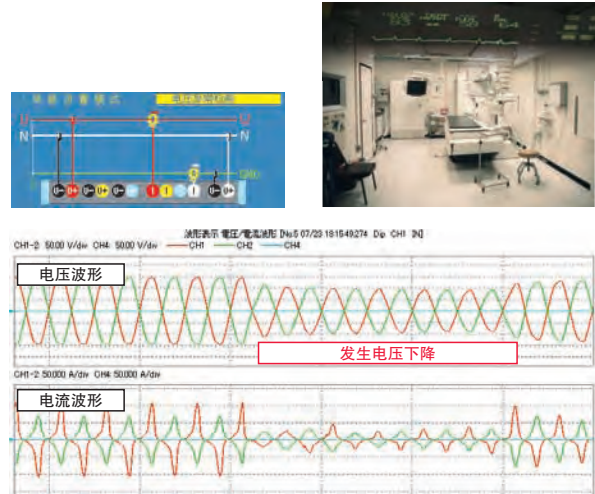
电压下降发生时的电压波形和电流波形
