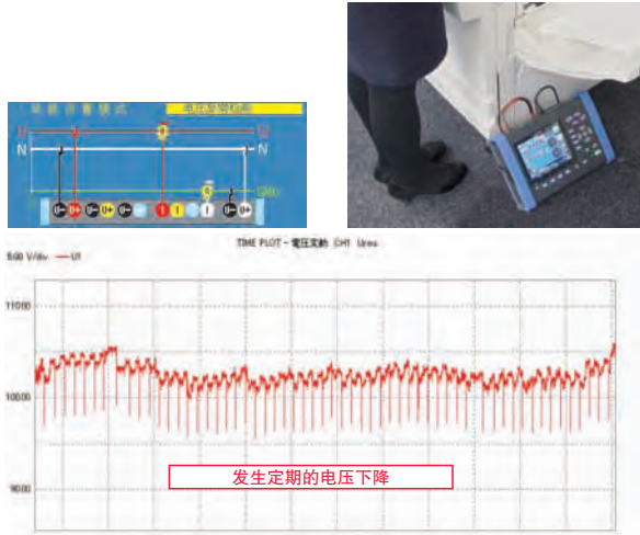
电压变动图
